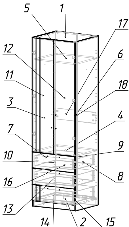
Рис.1 Схема сборки
